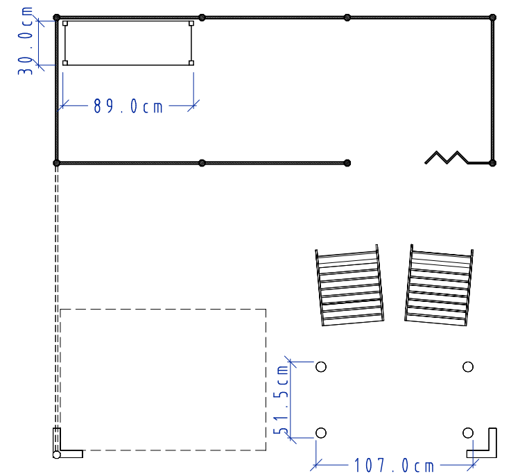
PLANIMETRIA (sezione h.60cm) PLAN (section h.60cm)
