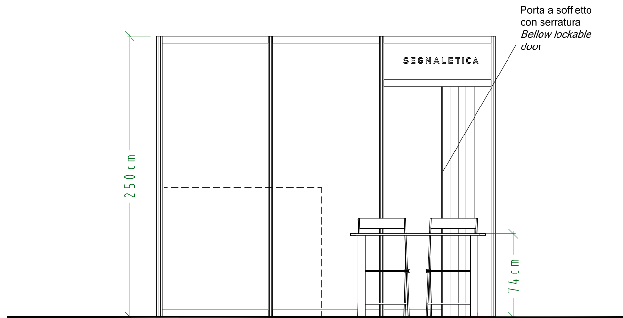
PROSPETTO/FRONT ELEVATION
